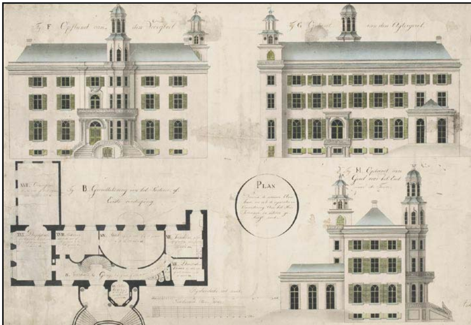
Niet uitgevoerd plan voor de verbouwing van het huis Sevenaer door architect J. Übbing, 1827 (coll. Gelders Archief, Archieven van de familie Van Nispen, inv.nr. 1773; foto Gelders Archief).
